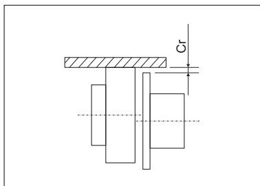
FIG. 27 (Allineamento e centraggio del giunto d'accoppiamento)
