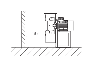
FIG. 15 (Aspirazione libera)
