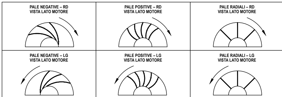
FIG. 3a Girante ventilatore centrifugo
