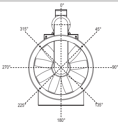
FIG. 10 (Posizione del motore su ventilatore assiale)
