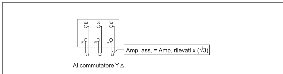
FIG. 31 (Equipaggiamento elettrico)
