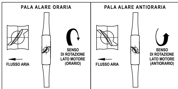
FIG. 3b Girante ventilatore assiale
