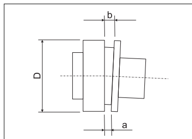
FIG. 28 (Allineamento e centraggio del giunto d'accoppiamento)
