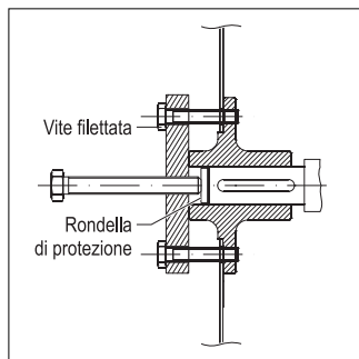
FIG. 18 (Smontaggio)
