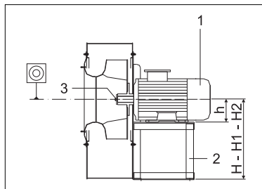
FIG. 16 (Montaggio del motore sulla sedia)
