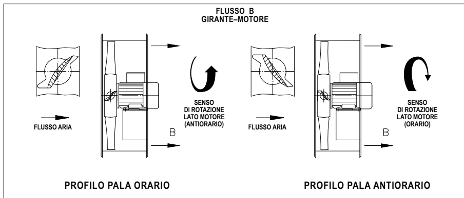
FIG. 20 (Flusso "B")
