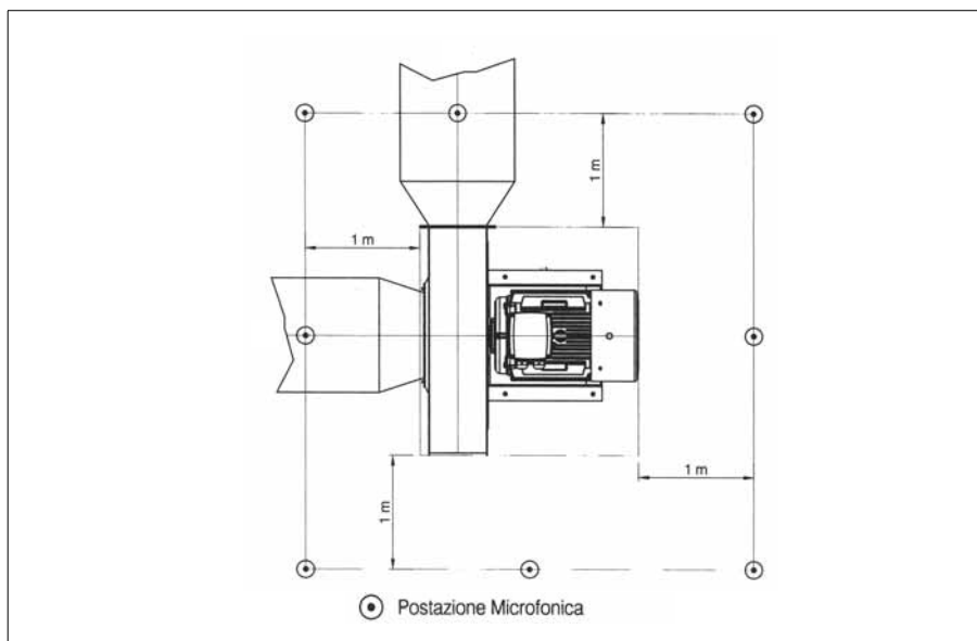
FIG. 35 (Rumore aereo)
