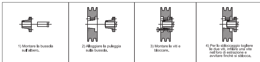
FIG. 25 (Montaggio delle pulegge)
