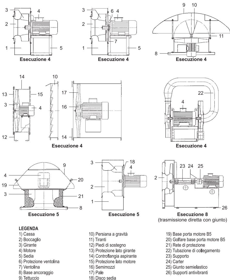
FIG. 4 (Esecuzione a trasmissione diretta)
