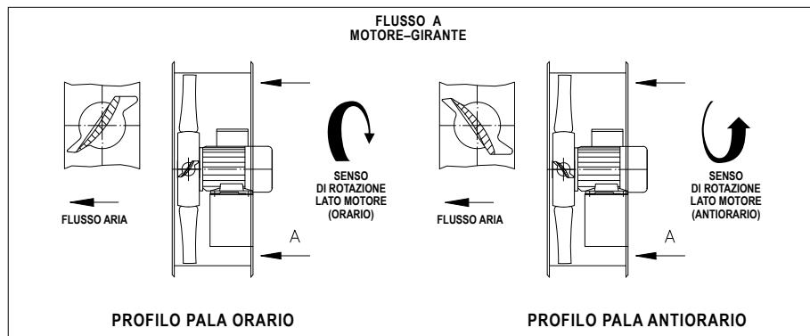
FIG. 19 (Flusso "A")
