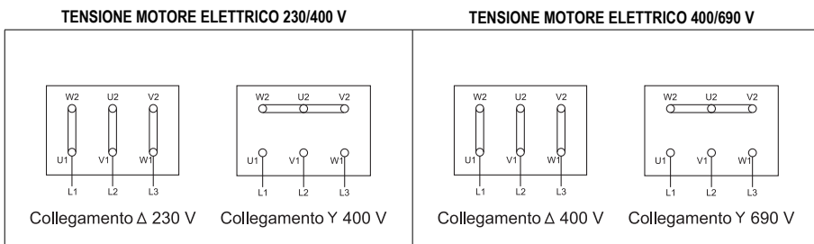
FIG. 29 (Motore elettrico 230/400 V)
