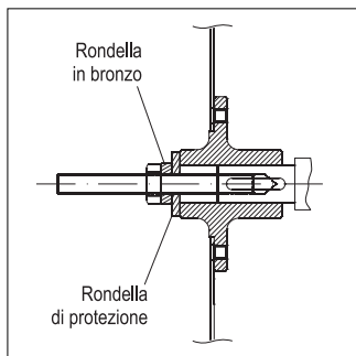
FIG. 17 (Montaggio)
