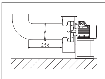
FIG. 14 (Collegamento a tubazioni)
