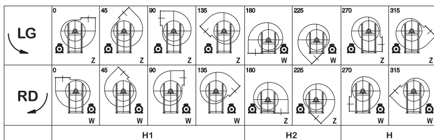
FIG. 9 (Orientamento con posizioni standard dei motori)
